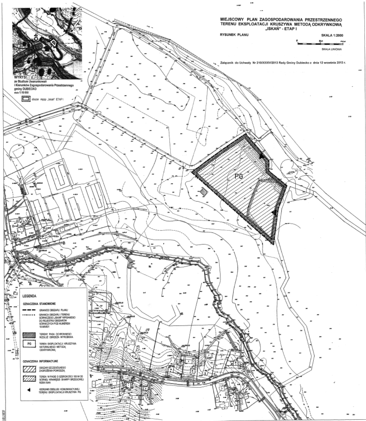
5517594 Mapa sytuacyjno-wysokościowa gm. Dubiecko obr. Iskań skala 1:2000 s. 8.119.07.06
